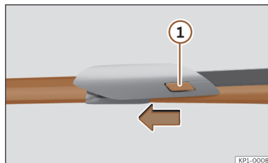
Afb. 207 Ruitenwisserbladen voorruit vervangen.
