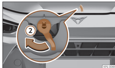
Afb. 220 Hendel onder de motorkap.
