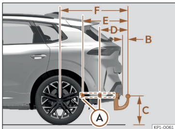
Afb. 199 Trekhaak: maten en bevestigingspunten.
