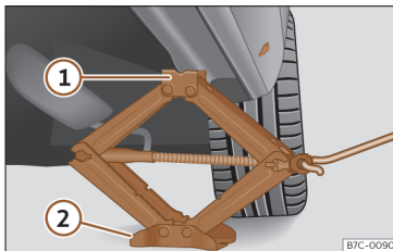
Afb. 243 Langsligger: plaatsing van de wagenkrik.
