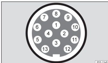
Afb. 195 Schematische weergave: toewijzing van de pinnen van het stopcontact voor de aanhangwagen.
