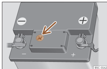
Afb. 232 Kijkglas aan de bovenzijde van de 12 volt-accu (schematische voorstelling).
