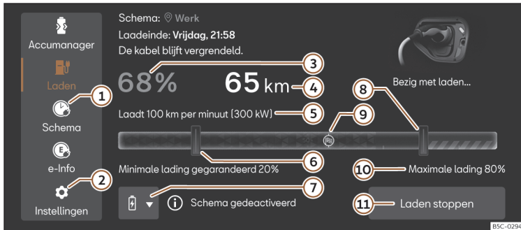
Afb. 64 In het infotainmentsysteem: hoofdmenu Laden.
