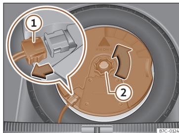
Afb. 238 In de bagageruimte: subwoofer uitbouwen.
