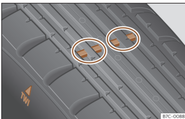
Afb. 235 Bandenprofiel: slijtagemerkttekens.
