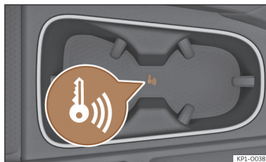
Afb. 115 In de middenconsole: noodstart.
