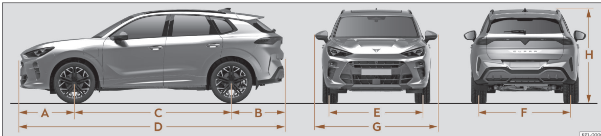
Afb. 249 Afmetingen
