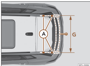
Afb. 200 Trekhaak: maten en bevestigingspunten.
