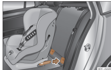
Afb. 42 Achterstoelen: plaatsing van het kinderzitje met ISOFIX-systeem.
