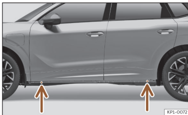
Afb. 242 Steunpunten voor de krik.
