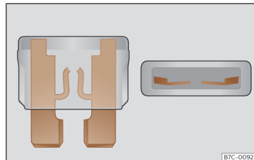
Afb. 218 Voorbeeld van een doorgebrande zekering.
