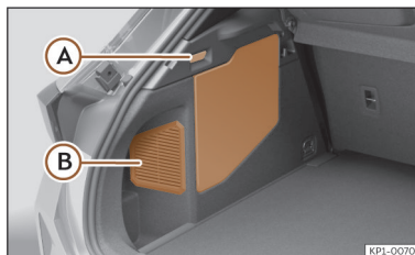
Afb. 231 Hybride wagens (PHEV): locatie van de accu in de bagageruimte
