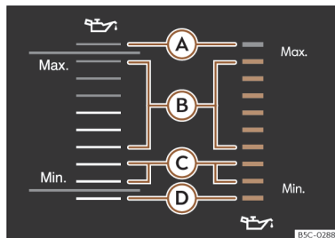
Afb. 230 Op het scherm van het infotainmentsysteem: mogelijke weergaven van de indicator van het motoroliepeil.
