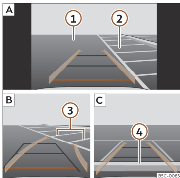
Afb. 165 Weergave op het scherm van het infotainmentsysteem: parkeren met de achteruitrijhulp.
