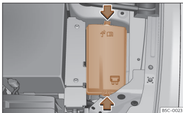
Afb. 218 In de motorruimte: deksel van de zekeringenhouder.
