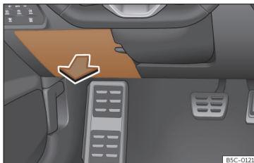
Afb. 217 In het dashboard aan bestuurderszijde: deksel van de zekeringenhouder.
