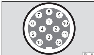
Afb. 198 Schematische weergave: toewijzing van de pinnen van het stopcontact voor de aanhangwagen.
