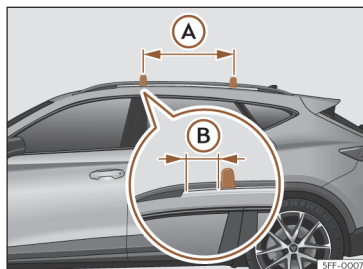
Afb. 197 Bevestigingspunten van de dwarsdragers voor het dakdragersysteem.
