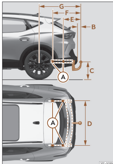
Afb. 202 Maten en bevestigingspunten voor het achteraf inbouwen van een trekhaak.
