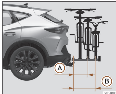
Afb. 201 Schematische voorstelling van de maximale overhang van de lading in een fietsendrager voor twee of drie fietsen.
