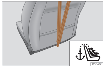
Afb. 40 Achterzijde van de rugleuning van de bijrijdersstoel: verankering voor de Top Tether-riem (niet in alle markten/versies beschikbaar).
