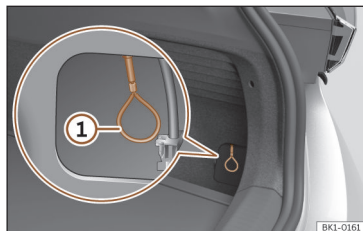
Afb. 62 Achter de afdekking: noodontgrendeling van de laadstekker.
