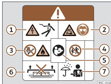
Afb. 52 Waarschuwingsschiltje op de hoogvoltageaccu.
