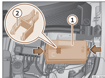
Afb. 192 In de voorruimte: deksel van de zekeringhouder.
