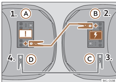
Afb. 185 Schakelschema van de startkabels.
