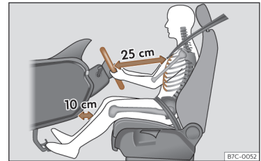
Afb. 15 De correcte afstand tussen de bestuurder en het stuurwiel moet minstens 25 cm (10 inch) bedragen.
