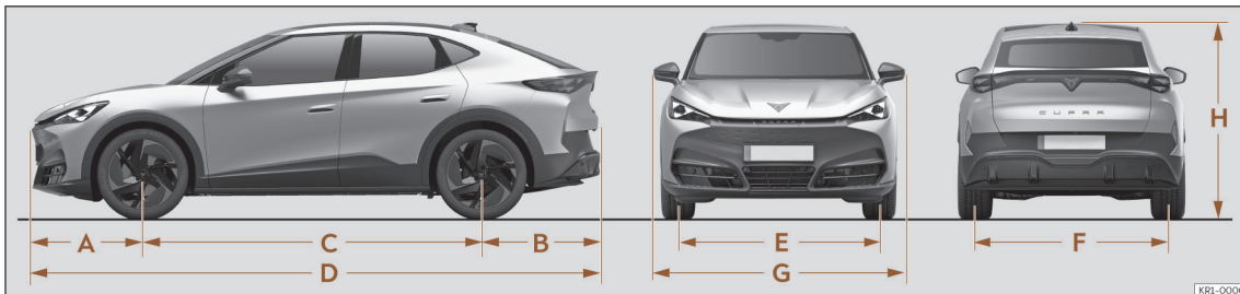
Afb. 212 Afmetingen
