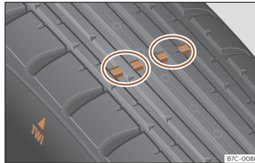
Afb. 201 Bandenprofiel: slijtagemerkttekens.
