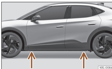
Afb. 206 Steunpunten voor de krik.
