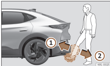
Afb. 79 Achterklep sensorgestuurd openen (Easy Open).
