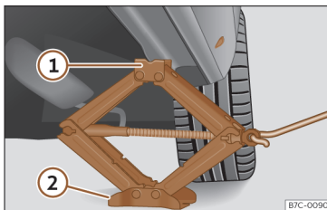
Afb. 207 Langsligger: plaatsing van de wagenkrik.
