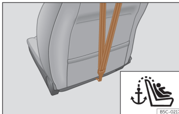
Afb. 43 Achterzijde van de rugleuning van de bijrijdersstoel: verankerung voor de Top Tether-riem (niet in alle markten beschikbaar).
