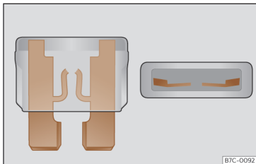
Afb. 214 Voorbeeld van een doorgebrande zekering.
