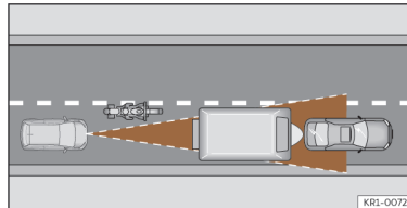
Afb. 141 Motorrijder die voor u rijdt, buiten de actieradius van de radarsensor.
