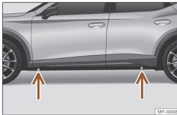
Afb. 238 Steunpunten voor de krik.
