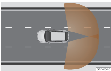
Afb. 132 Detectiegebieden van de sensoren.
