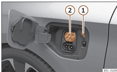
Afb. 59 Achter de laadklep van de accu linksvoor: laadcontactdoos.
