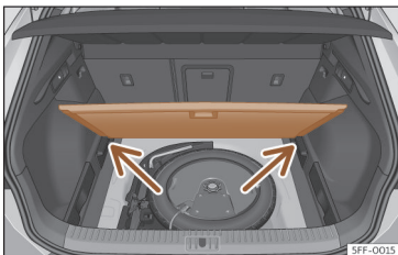
Afb. 187 Verstelbare bodem van de bagageruimte: schuine stand.
