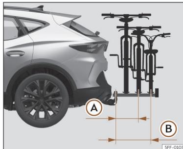
Afb. 198 Schematische voorstelling van de maximale overhang van de lading in een fietsendrager voor twee of drie fietsen.
