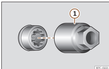
Afb. 236 Wielbout met diefstalbeveiliging, voorzien van dop en adapter.
