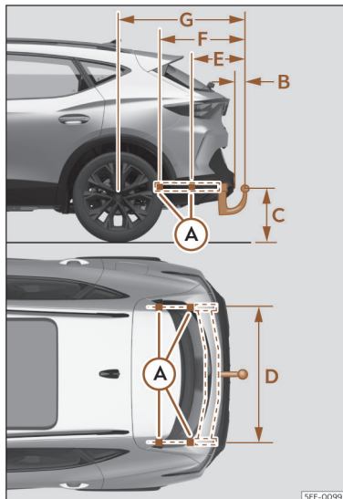
Afb. 199 Maten en bevestigingspunten voor het achteraf inbouwen van een trekhaak.
