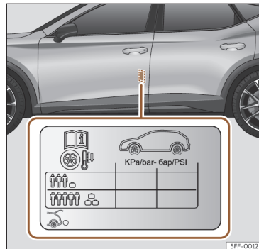
Afb. 230 Plaats van de sticker van de bandenspanningen.
