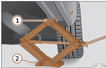
Afb. 239 Langsligger: plaatsing van de wagenkrik.
